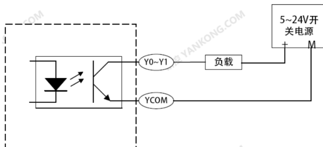
Y0~Y1 接成 sinking 型输出
