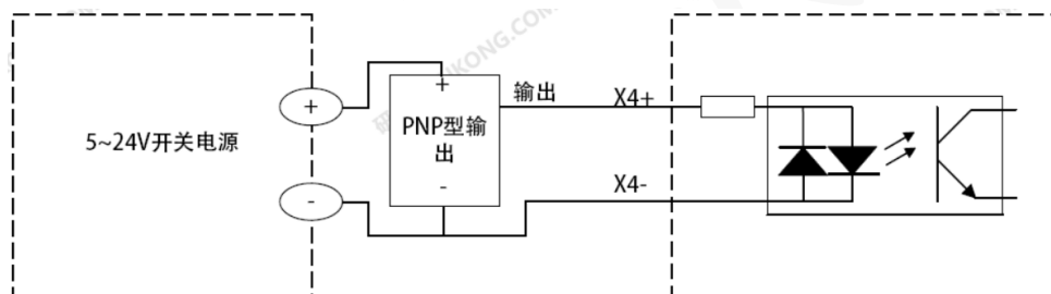
差分信号 X4 接入到 PNP 输出
