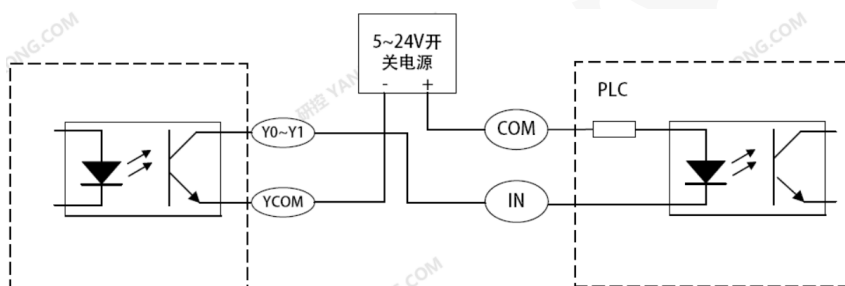
将 Y0~Y1 接成 sinking 型输出，连接到 PLC
