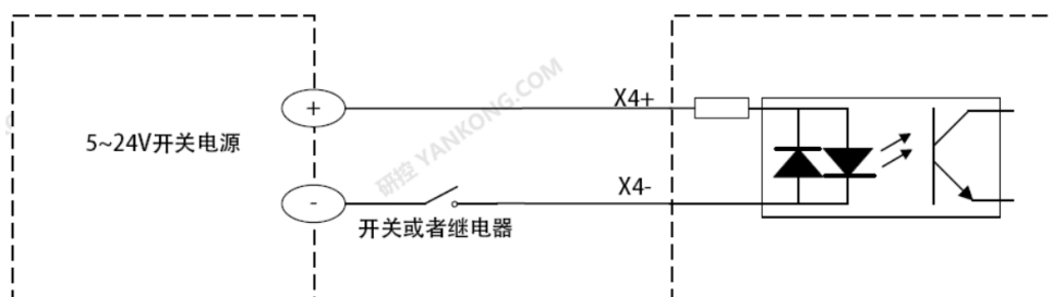
差分信号 X4 接入到开关或继电器
