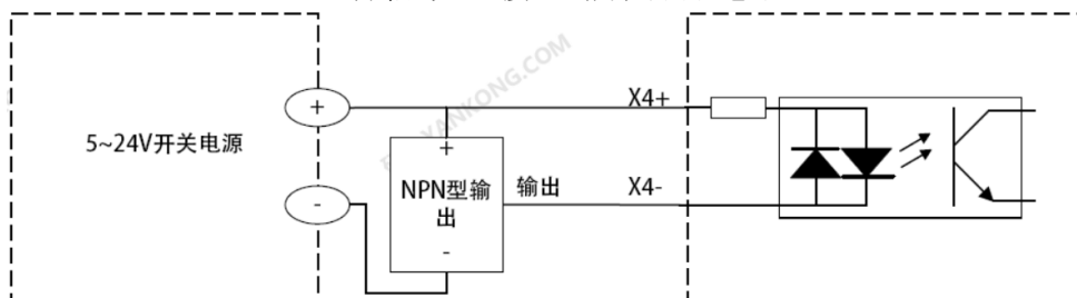
差分信号 X4 接入到 NPN 输出
