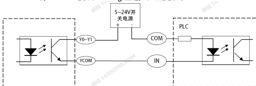
将 Y0~Y1 接成 sourcing 型输出，连接到 PLC
