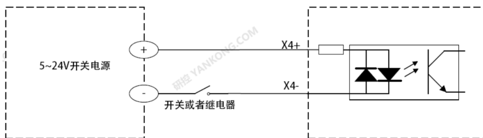
差分信号 X4 接入到开关或继电器
