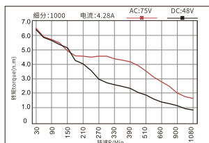
电机型号:YK86HB118-06A
