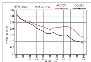
电机型号:YK86HB65-04A
