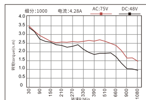
电机型号:YK86HB80-04A
