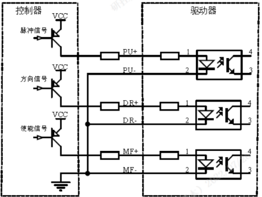
共阴极接法
