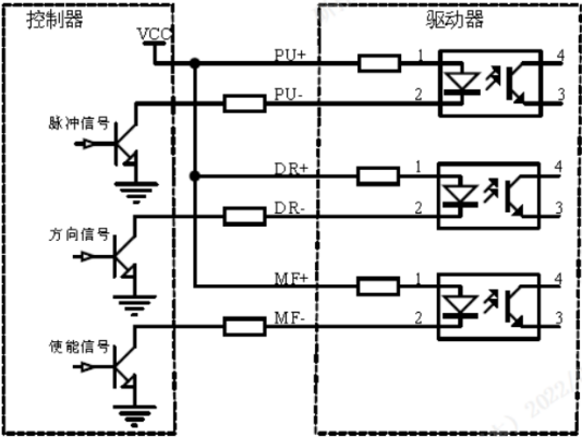
共阳极接法
