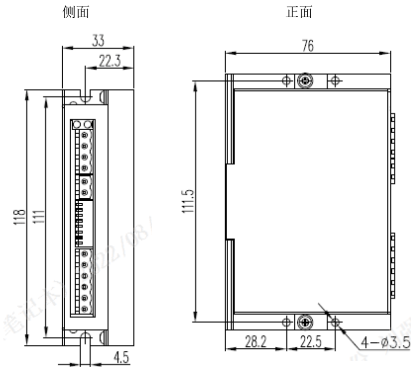
安装尺寸图 (单位: mm)
