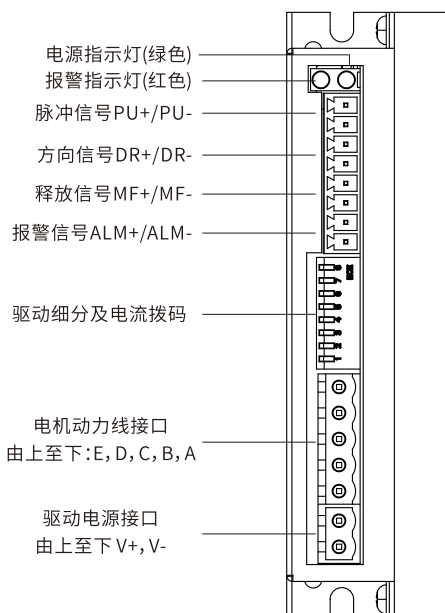
驱动器接线示意图
