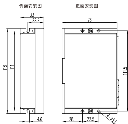
安装尺寸(单位:mm)
