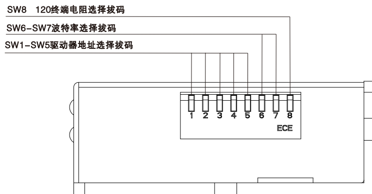
驱动器顶部接线示意图
