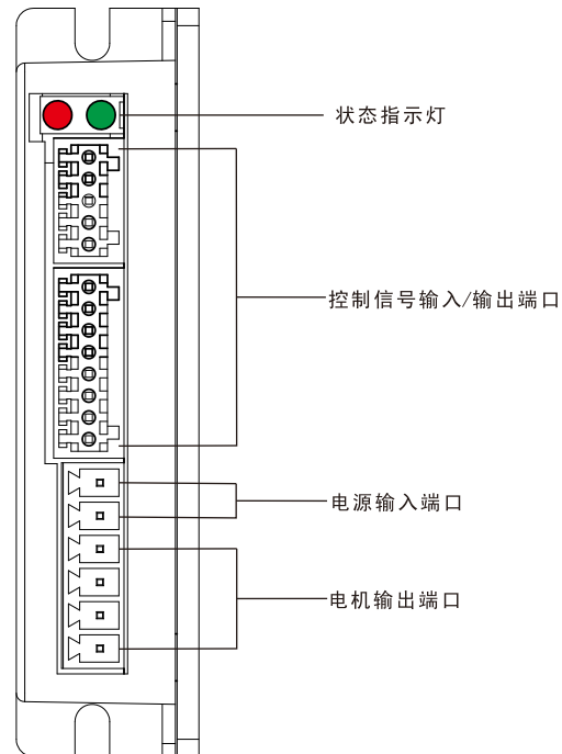
驱动器侧面接线示意图
