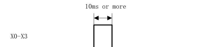
X0-X3 时序图
