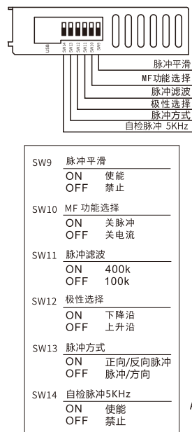
DIP开关功能设定说明
