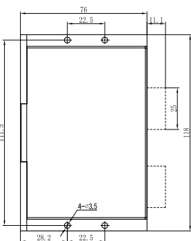
正面安装图
