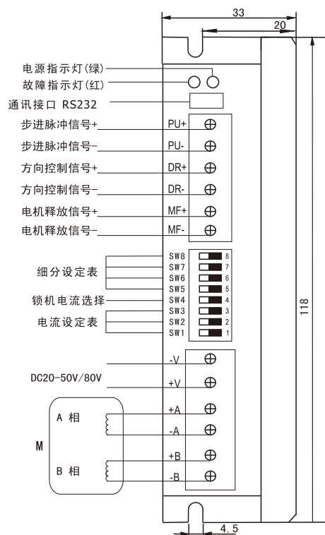
驱动器接线示意图
