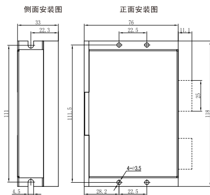
安装尺寸(单位:mm)
