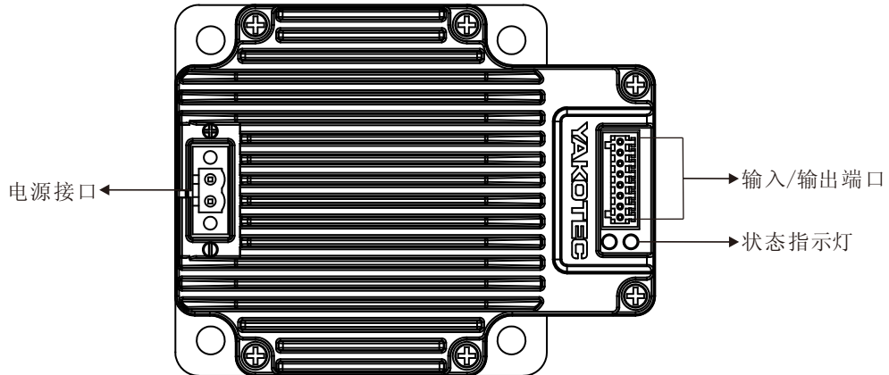
接线示意图
