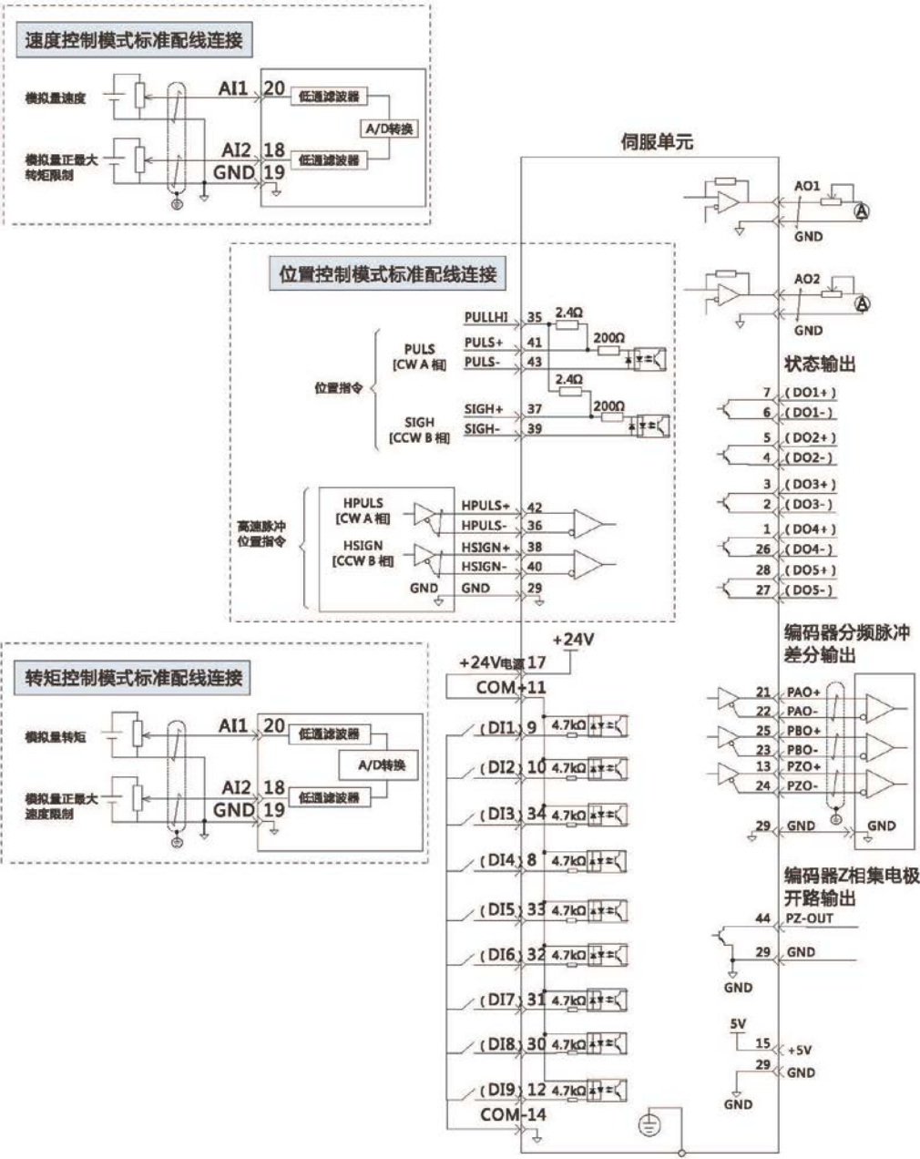
图 3-2 控制模式总图
