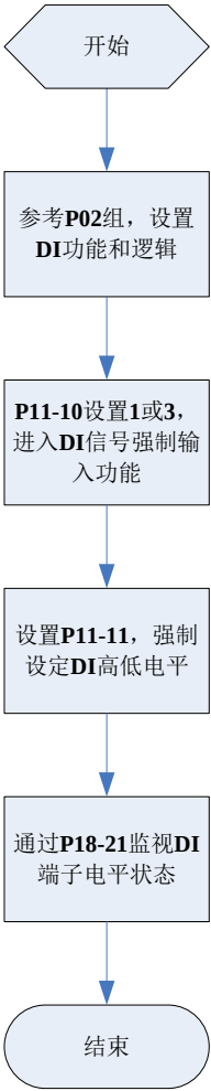
图 5-1 DI 信号强制输入设定步骤示意图
