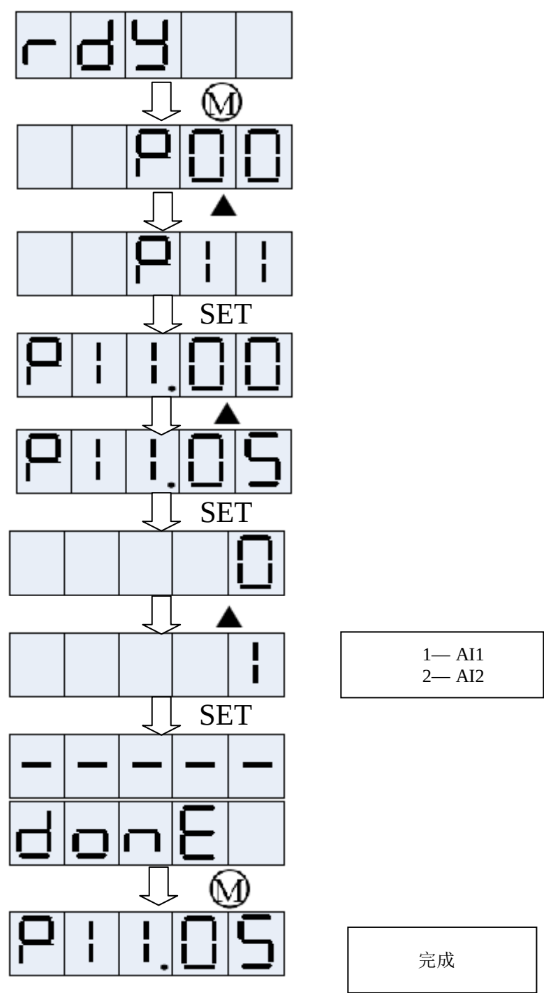
模拟量指令偏移量调整流程图
