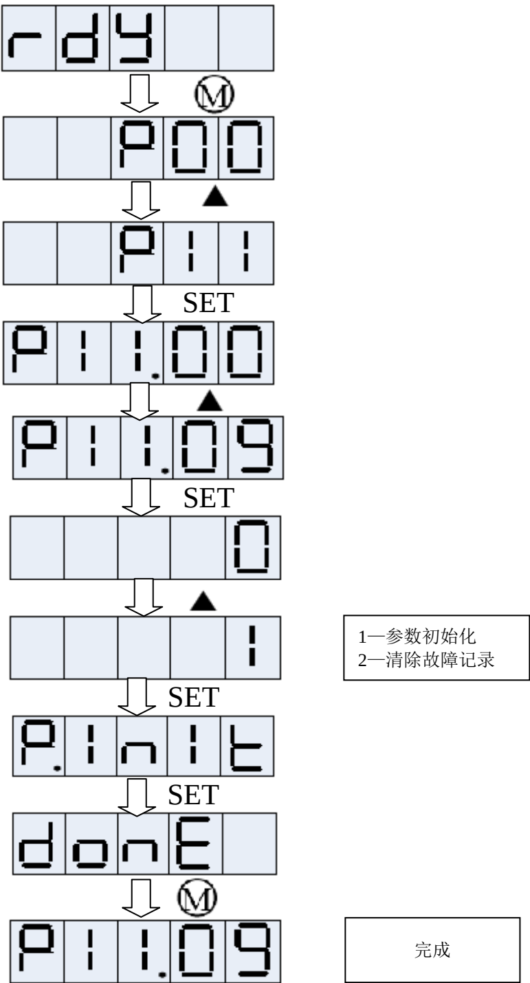
参数初始化流程图
