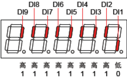
图 5-2 P18-21 对应 DI 电平状态说明
