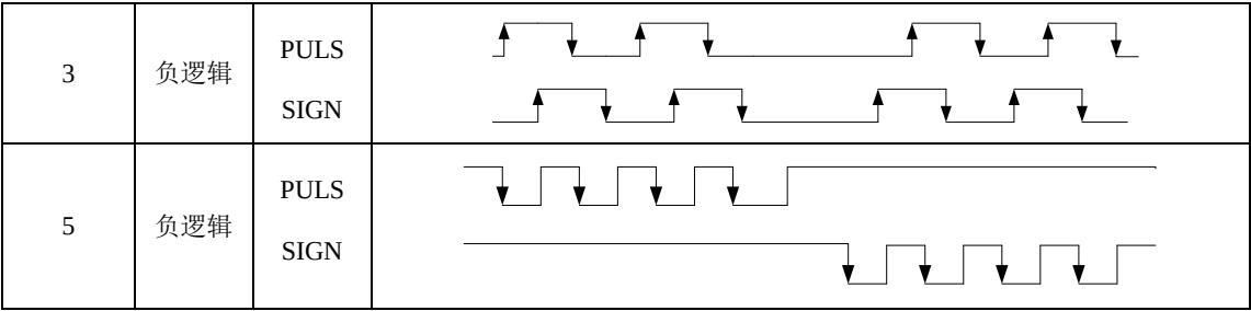
d) 脉冲禁止输入
