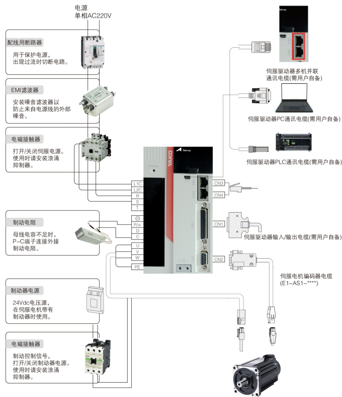
图 3-1 系统结构图
