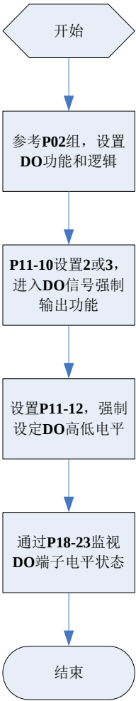
图 5-3 DO 信号强制输出设定步骤示意图
