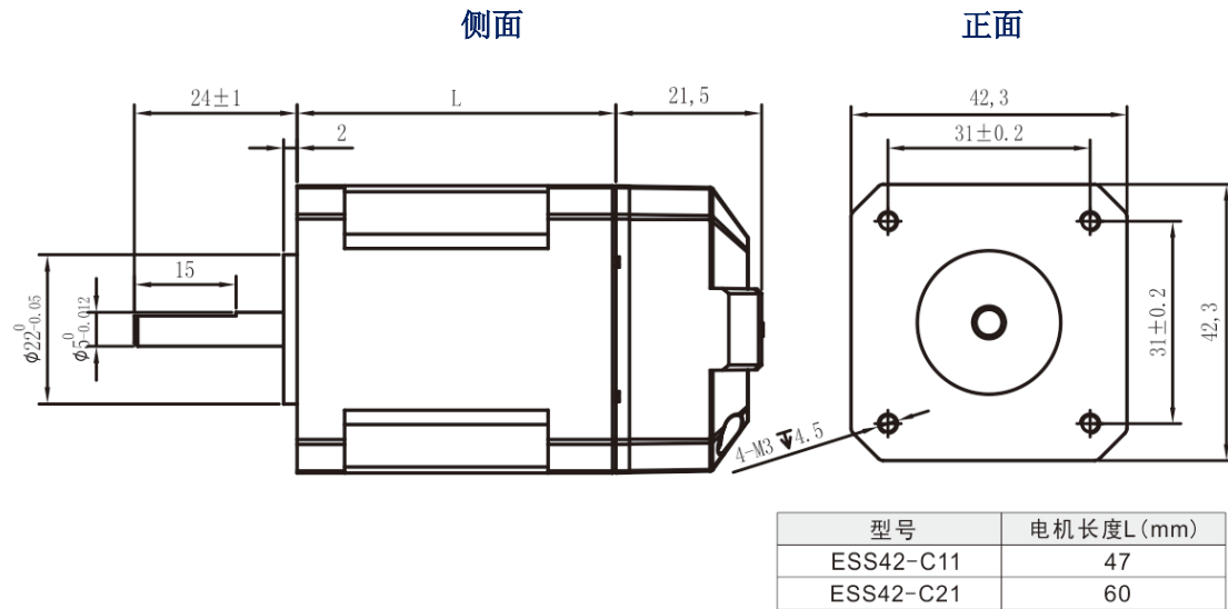
安装尺寸图 (单位: mm)
